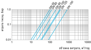
Рис. 3.1. Графік втрати тиску лічильників WPD
