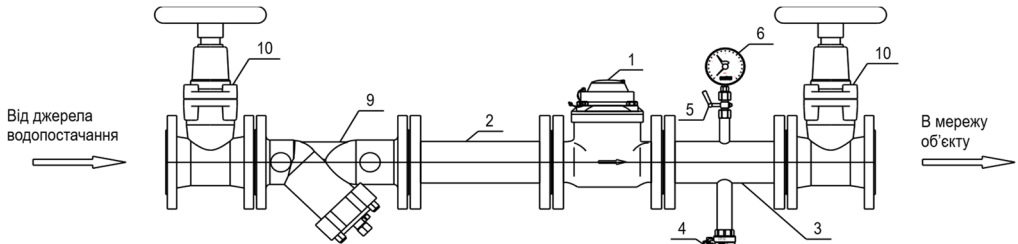
Рис. 2. Рекомендована схема встановлення лічильника
